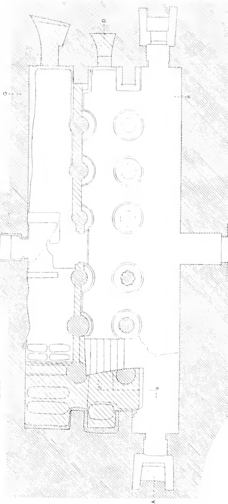
PLAN.
